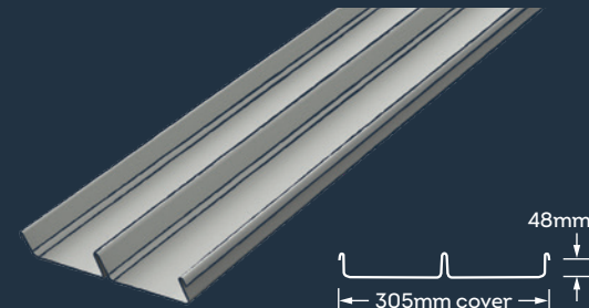
Shadowline® 305 (WA variant)
